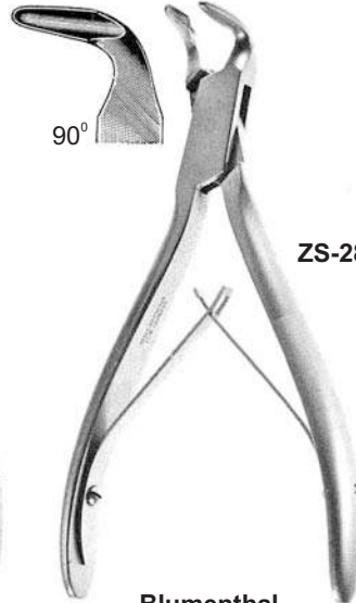
Blumenthal 90°, 16 cm 6 1/4" ZS-28-237-090
